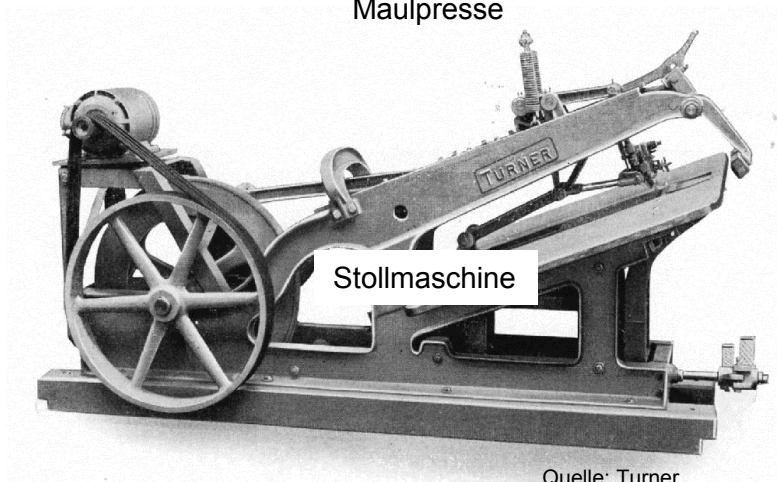
Maulpresse
