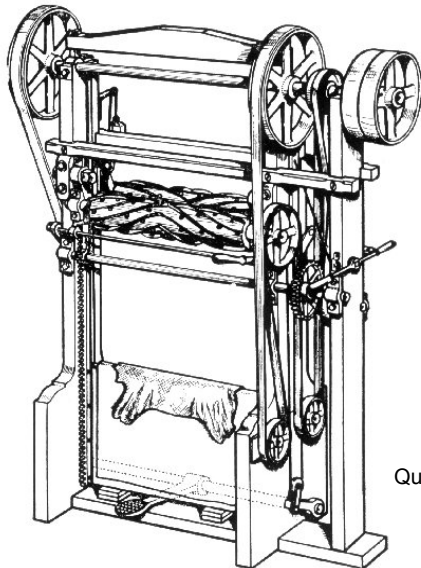
Eintisch-Ausreckmaschine von Vaughn Eintisch-Ausreckmaschine von Vaughn (Strecken und Enthaaren)
