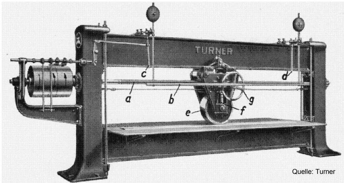
Karrenwalze mit Transmissionsantrieb zur Verdichtung von Sohlenleder
