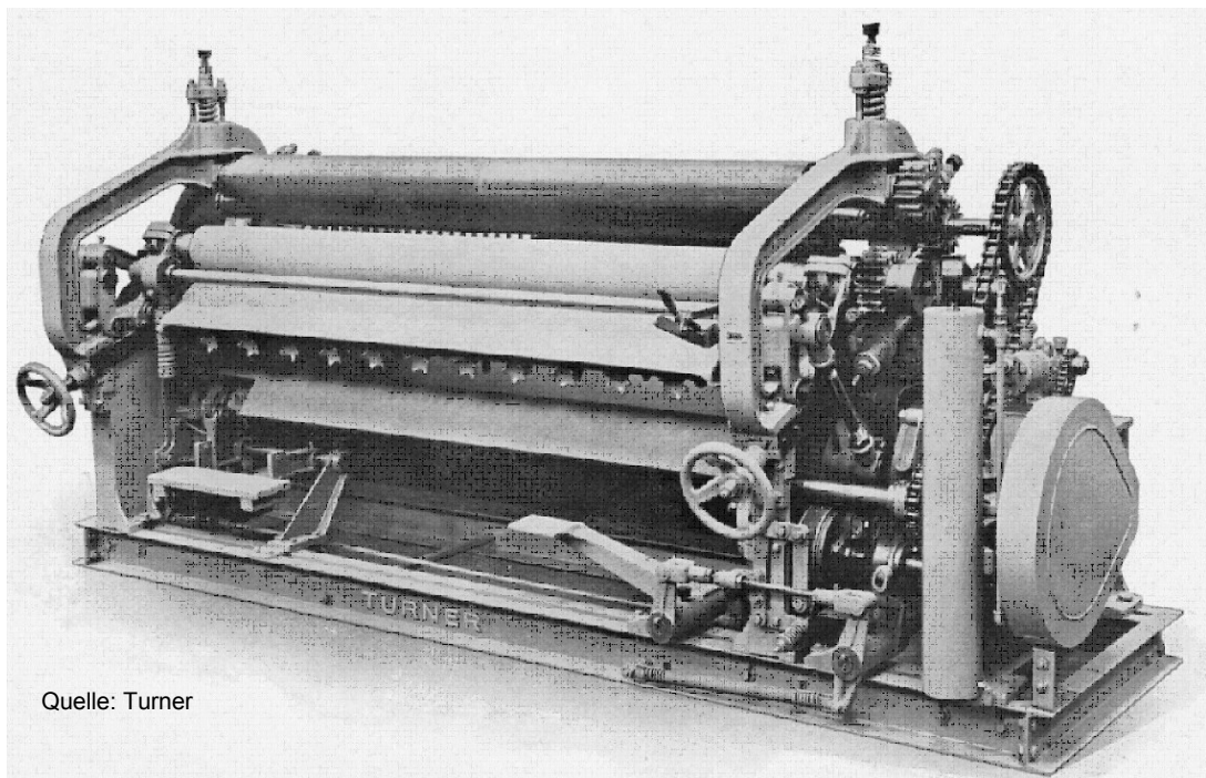
Pneumatische Entfleischmaschine für nasse Häute 2700 mm
