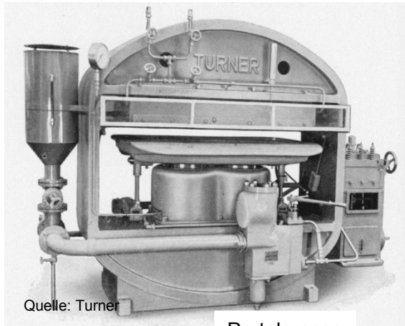
Portalpresse
