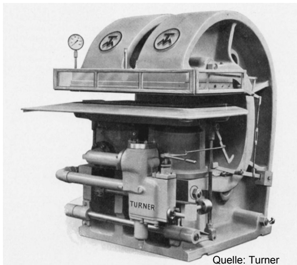
Maulpresse
