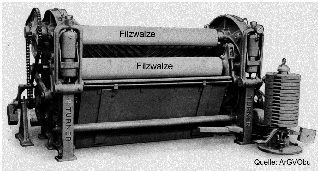
Abwelkpresse zum Entwässern von Leder um Nachrocknung zu verkürzen. (2700 mm)
