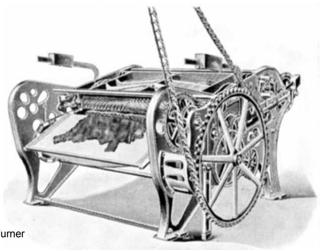
Reihentisch-Ausreckmaschine von Turner Reihentisch-Ausreckmaschine von Turner (Strecken und Enthaaren)
