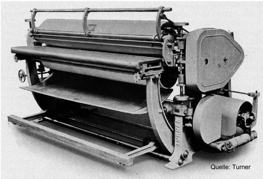
Krispelmaschine
