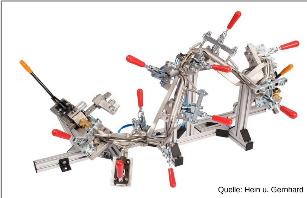
Dampf-Rohrbiegeform
