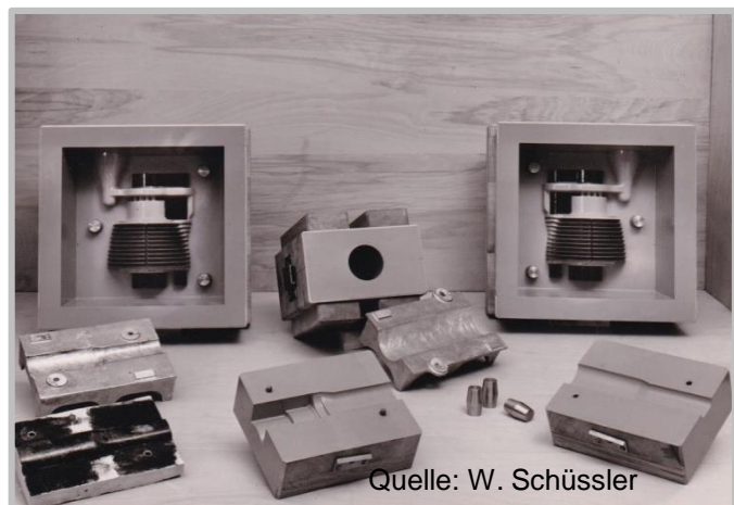
Rippenzylinder Kernform
