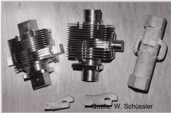
Rippenzylinder Croning
