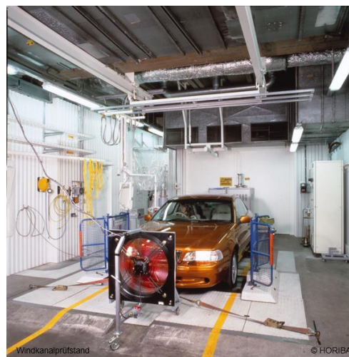
Rollen- und Windkanalprüfstand
