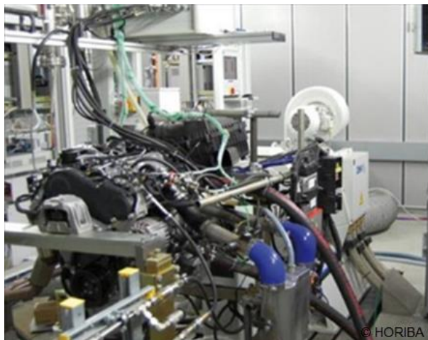
Motorenprüfstand
