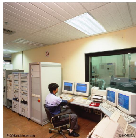
TestCenter: Prüfstandsteuerung – Schalt- und Bedienungszentrale (alt)
