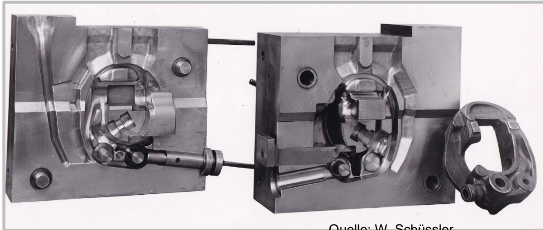
Achsschenkel-Stahl-Kokille
