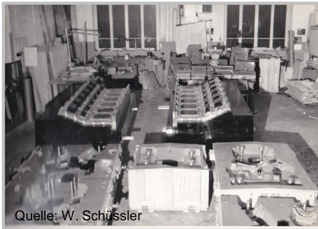
Kernkasten f. kleinen Schiffsmotor
