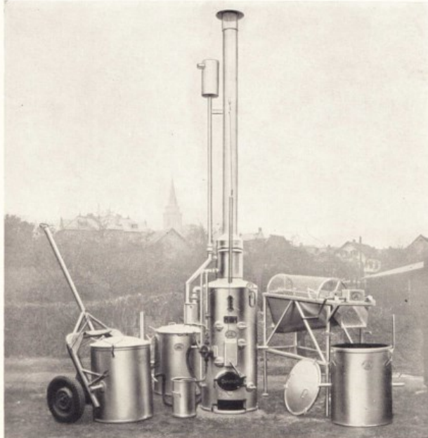
Dämpfkolonne Fig. 1
