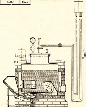
Fig. 317 — Schnitt
