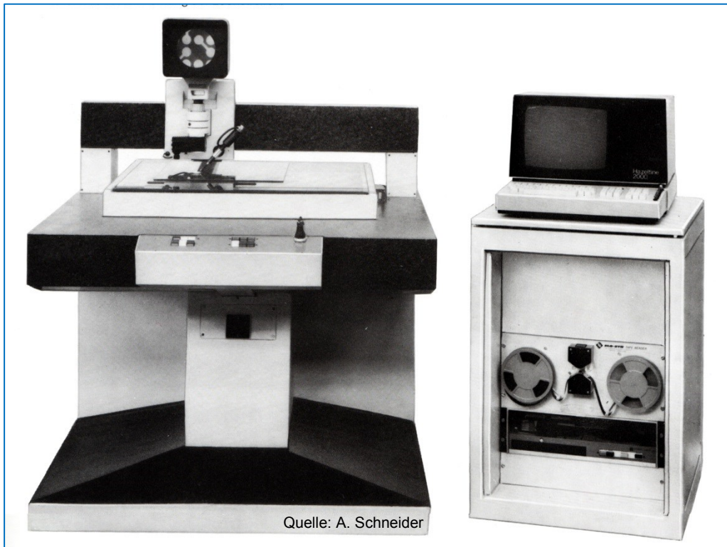
NC-Programmierplatz
