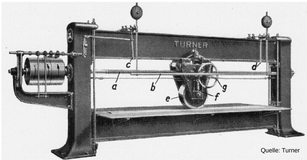
Karrenwalze mit Transmissionsantrieb zur Verdichtung von Sohlenleder
