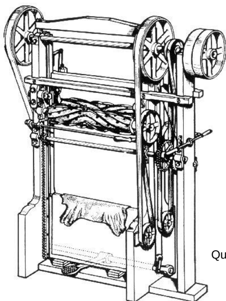
Eintisch-Ausreckmaschine von Vaughn Eintisch-Ausreckmaschine von Vaugh (Strecken und Enthaaren)
