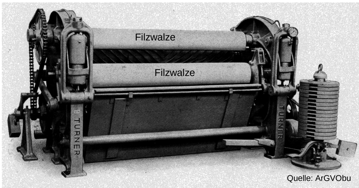
Abwelkpresse zum Entwässern von Leder um Nachtrocknung zu verkürzen. (2700 mm)
